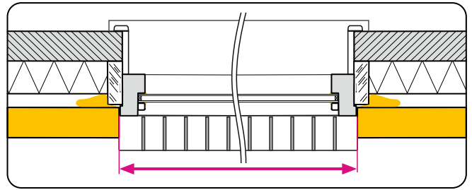
Doorsnede horizontaal
