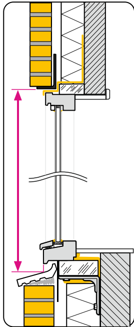
Doorsnede verticaal
